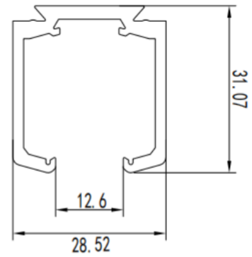
标准轨道：2201截面图
