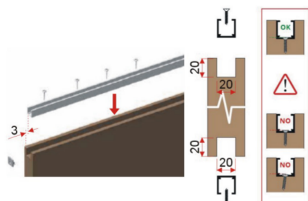
第一步：门板开槽放入铝条并用螺丝固定
