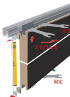
第五步：用扳手调节门高度，并保持门的水平，最后锁死固定
