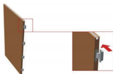
第六步：安装门板连接暗铰
