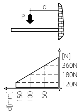
荷载能力图
