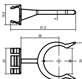
铝型材卡扣 P.A457.36.55
