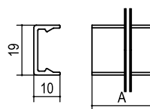
铝型材踢脚线 JS08.
