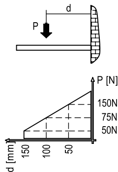
荷载能力图
