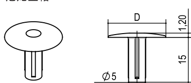
尼龙盖帽
